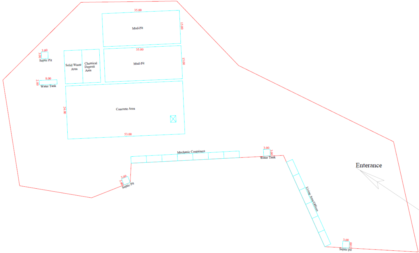
Şekil 2-12. ZDM-3 Kuyu Lokasyonu Yerleşim Planı 7
