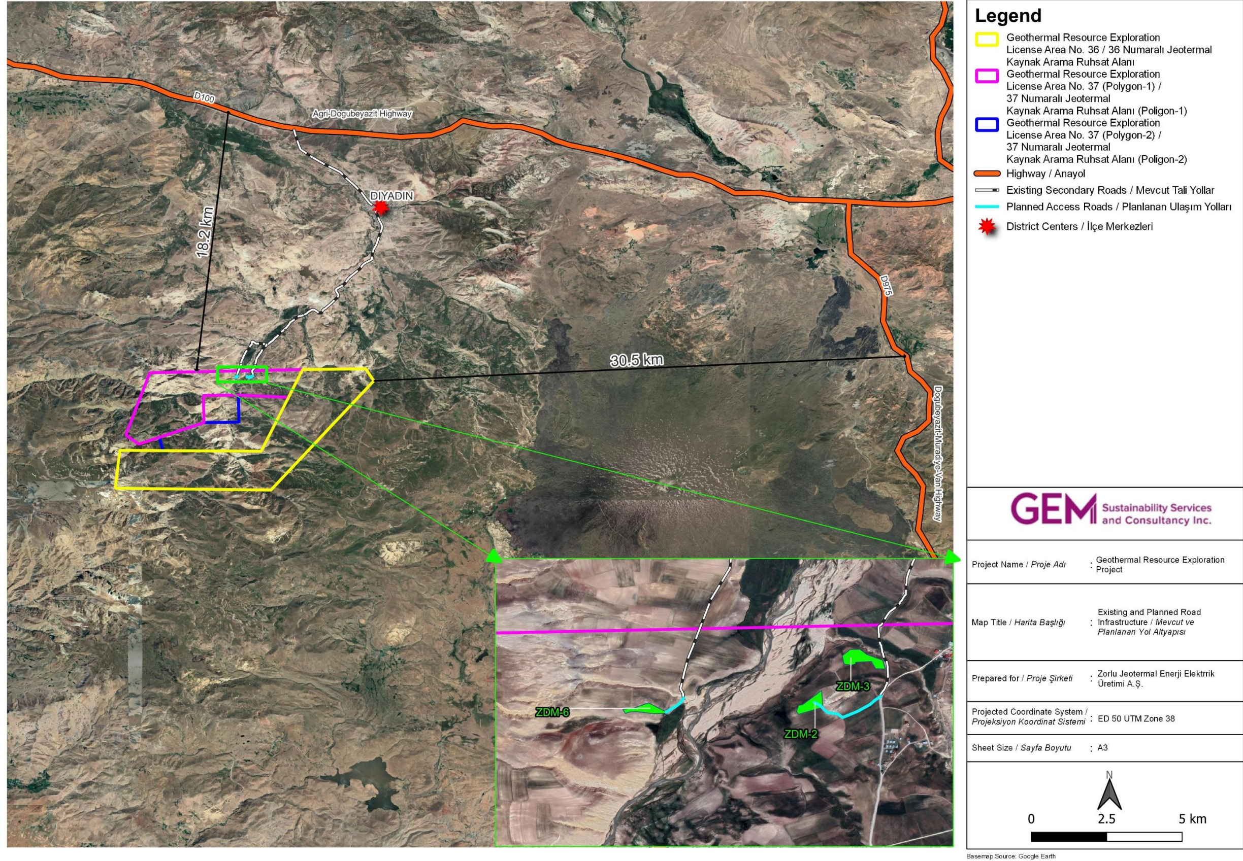
Şekil 2-7. Kuyu Yerlerine Planlanan Erişim Yolları
