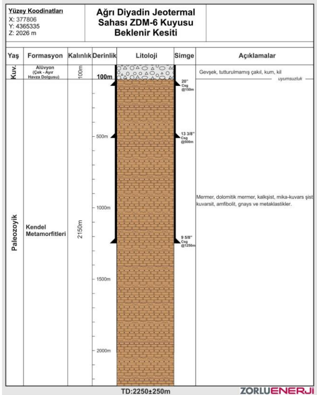
Şekil 2-15. ZDM-6 Kuyusunun Beklenir Kuyu Kesiti
