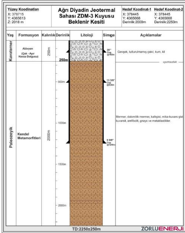
Şekil 2-13. ZDM-3 Kuyusunun Beklenir Kuyu Kesiti
