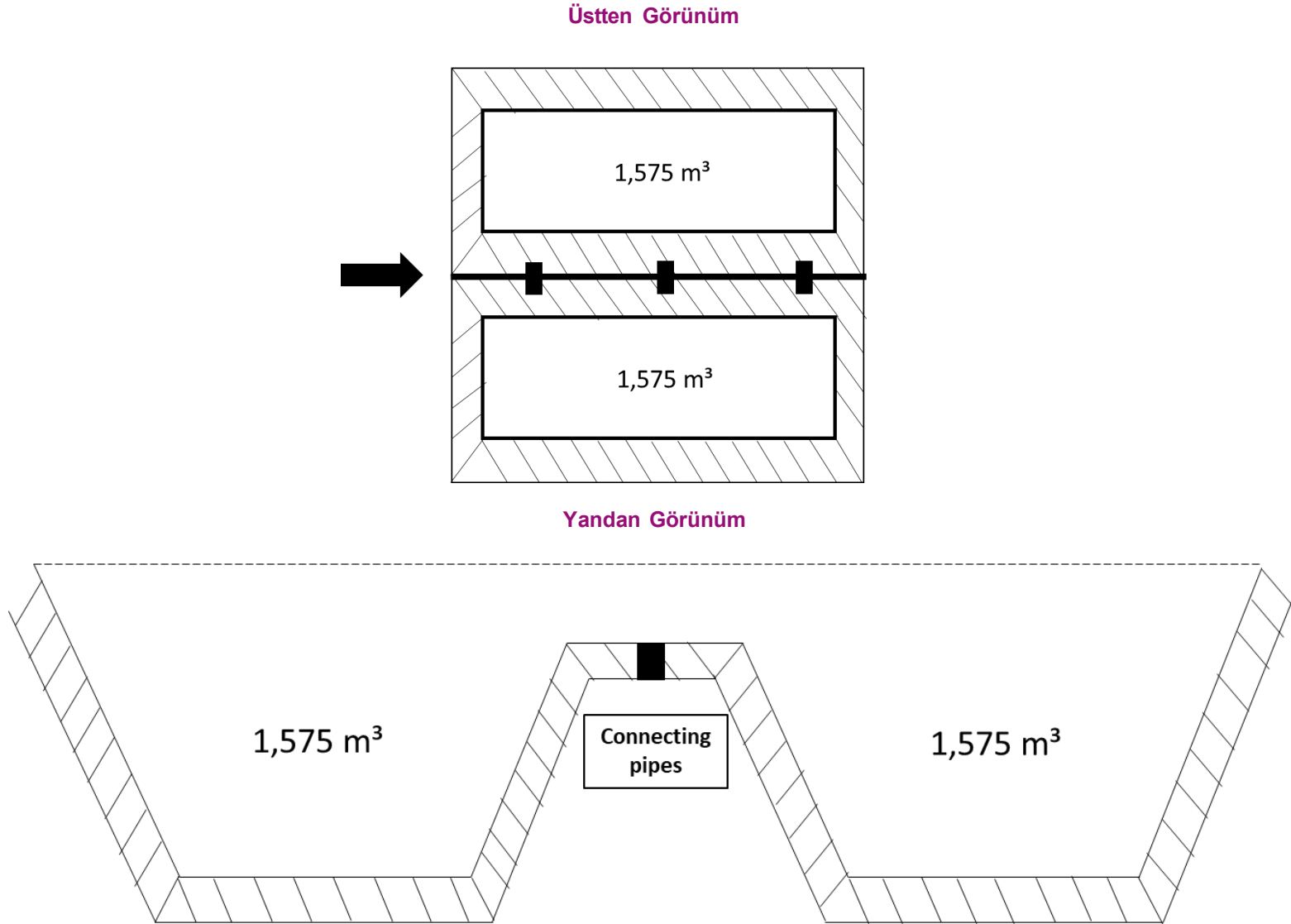
Şekil 2-11. Çamur Havuzlarının Üstten ve Yandan Görünümleri
