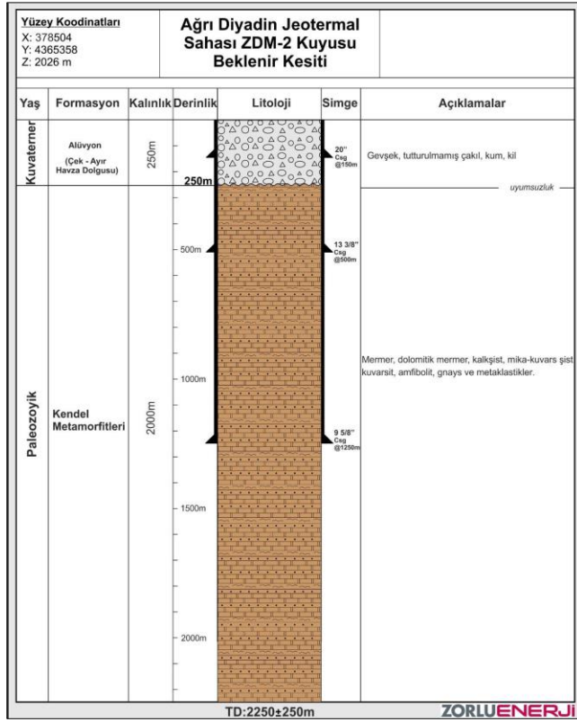
Şekil 2-14. ZDM-2 Kuyusunun Beklenir Kuyu Kesiti
